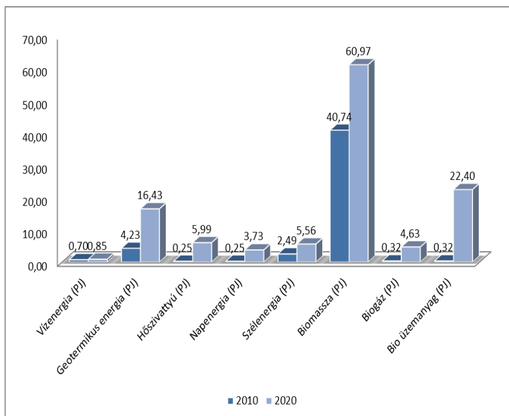
A megújuló energiahordozók megoszlása 2010-ben és a 2020-ra elérendő célok Magyarországon (6. ábra)
