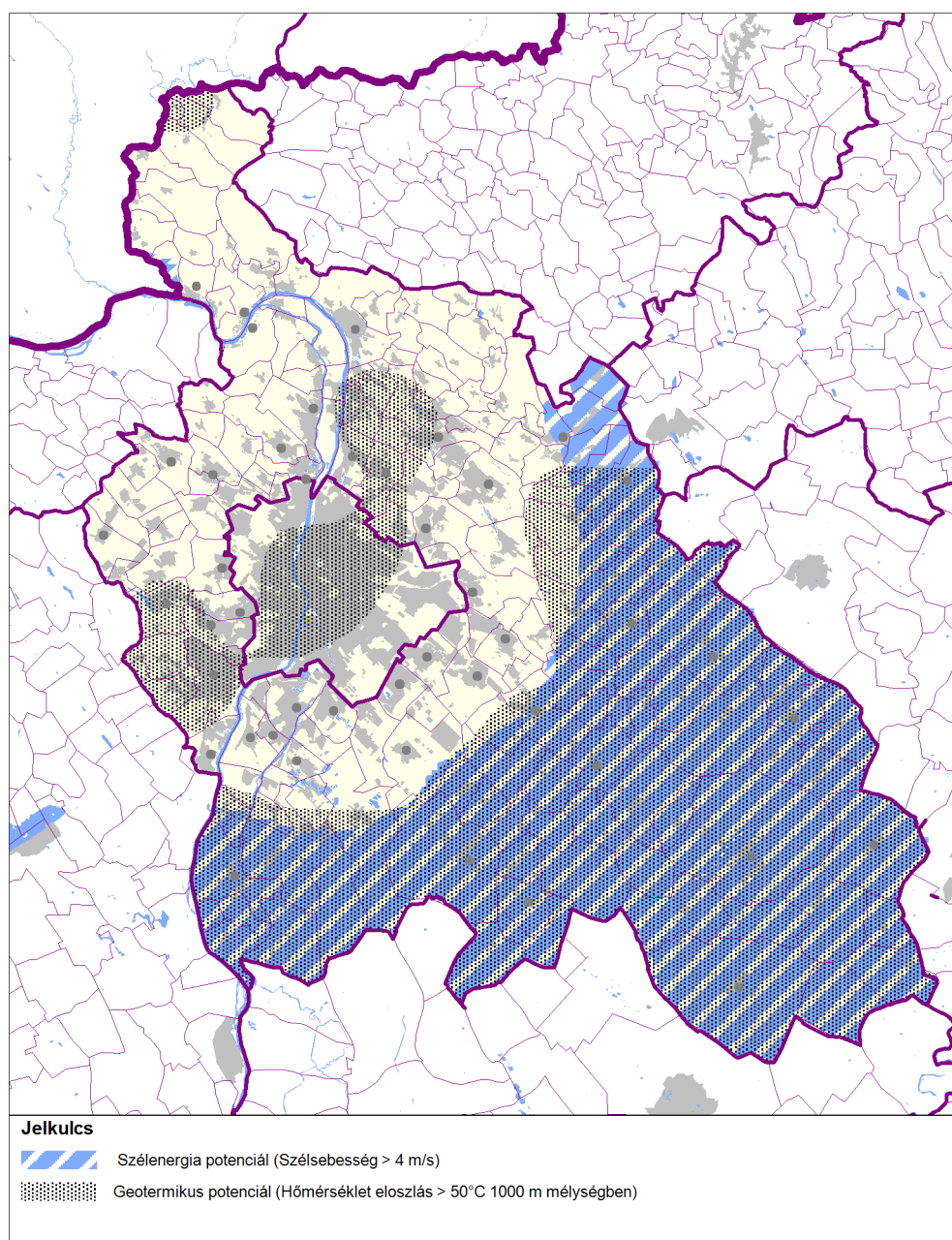
Szél és geotermikus energia potenciál Pest megyében (23. ábra)
