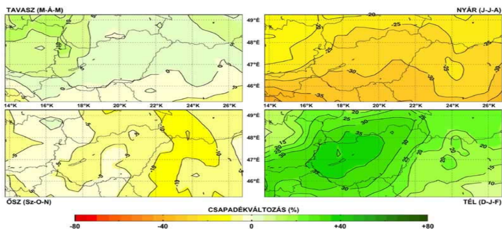
1.6. ábra - Évszakai csapadékváltozás (%) a Kárpát-medence térségére a PRUDENCE projektben alkalmazott európai regionális (50 km-es rácsfelbontású) éghajlati modellek eredményei alapján a 2071–2100 időszakra
