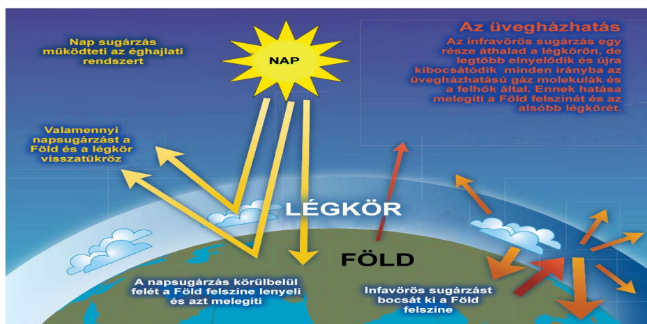
1.1. ábra – Az üvegházhatás egyszerűsített folyamata – Forrás: IPCC 4. értékelő jelentés, 2007
