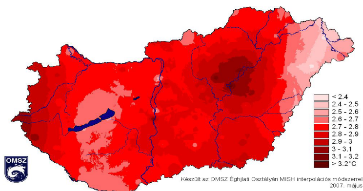
1.3. ábra – A nyári maximumhőmérséklet változása 1975-2004 – Forrás: OMSZ
