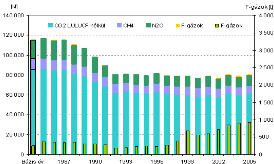
3.1. ábra – Üvegházhatású gázok kibocsátásának változása (CO 2 egyenértékben) nyelők által történő szén-dioxid megkötés nélkül Forrás: Nemzeti ÜHG Kibocsátási Leltár, 2007.
