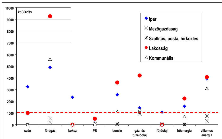
3.5. ábra – Az egyes szektorok energetikai eredetű CO 2 kibocsátásai energiafajták szerint – Forrás: Energiagazdálkodási statisztikai évkönyv, 2005 alapján
