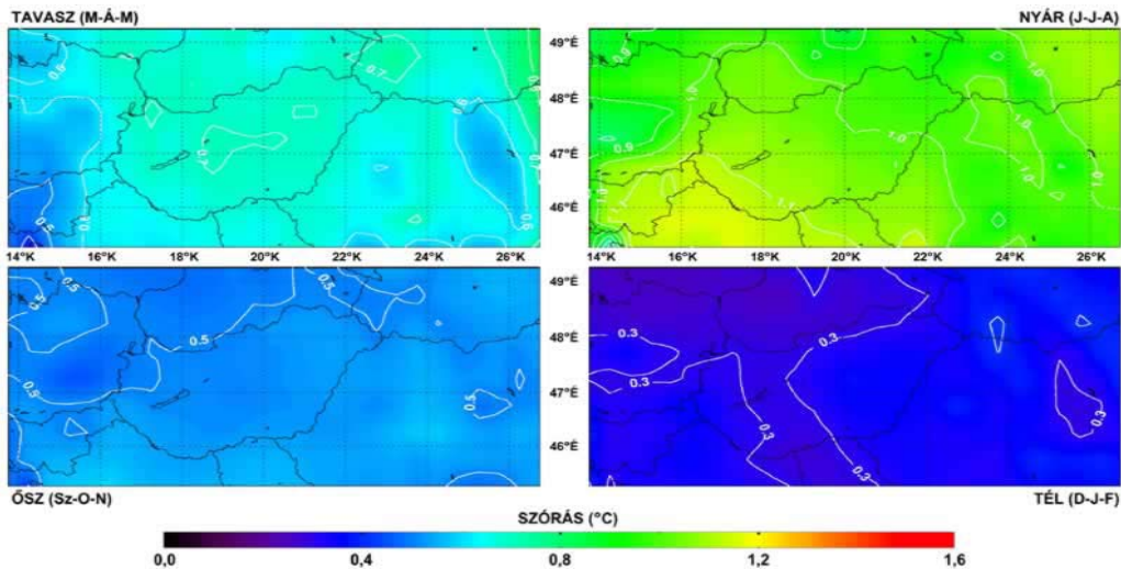
1.5 ábra - Az évszakai hőmérsékletváltozások szórása (°C) a Kárpát-medence térségére a PRUDENCE projektben alkalmazott európai regionális (50 km-es rácsfelbontású) éghajlati modell eredményei alapján a 2071–2100 időszakra
